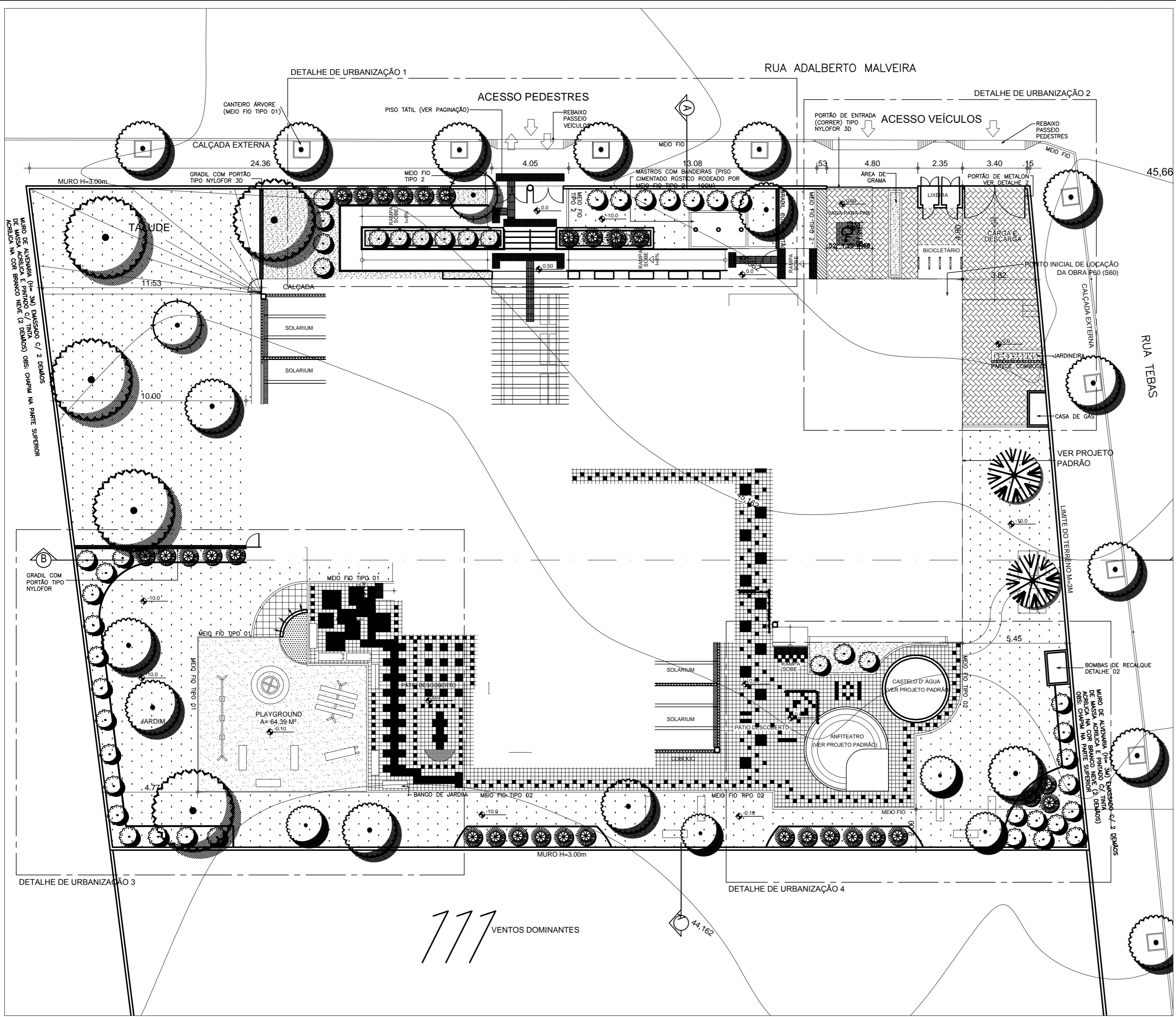
1 PLANTA GERAL DE PAISAGISMO ESC.: 1:150
